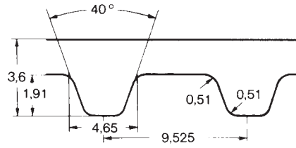
Type L (nur Mittelwerte nominal dimensions – mm)
