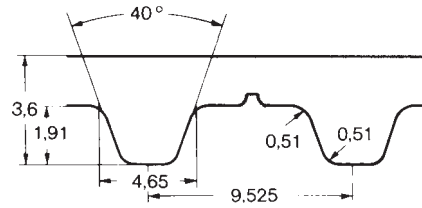
Type L (nur Mittelwerte nominal dimensions – mm)
