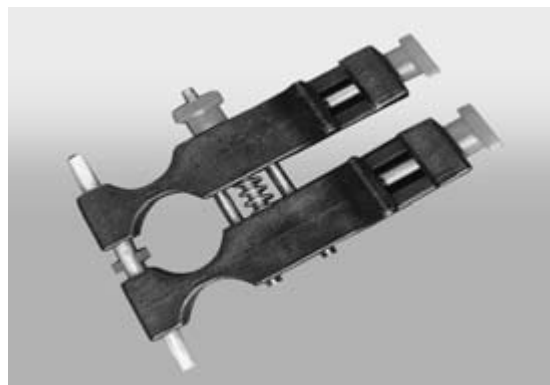
Miniführungszange R-8 für Rundriemen bis 8 mm Mini pliers R-8 for round belts up to 8 mm Euro 136,90
